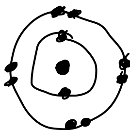
sodium ion
